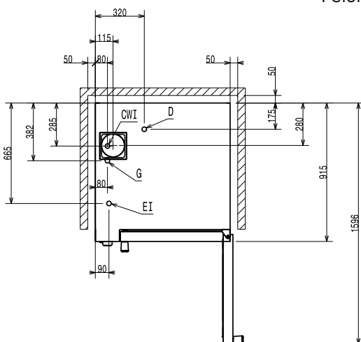
Felülnézet
